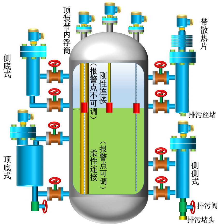
安装示意图
