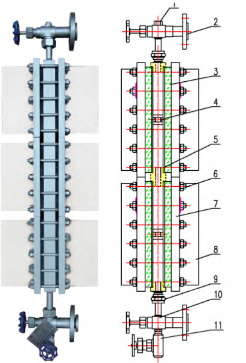
1.放空丝堵 2.连接法兰 3.玻璃板玻璃 4.玻璃板芯 5.垫片 6.紧固件 7.压盖 8.防霜玻璃 9.连接接头 10.考克阀体 11.排污阀
