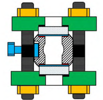
大口径透射式双色玻璃板液位计
