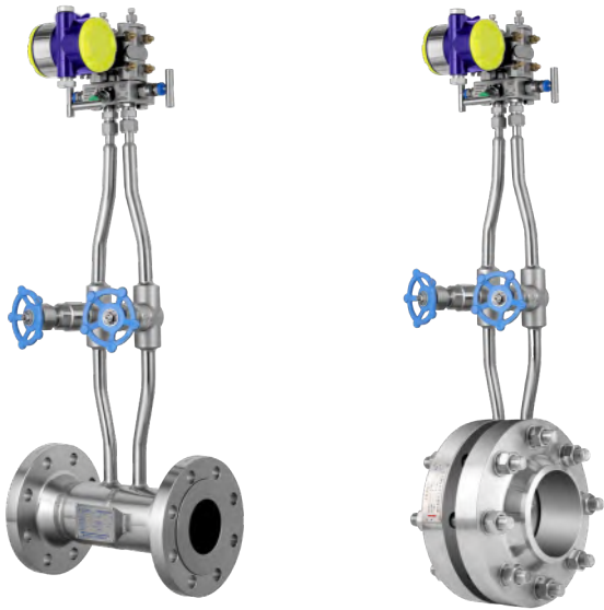
管道法兰式
