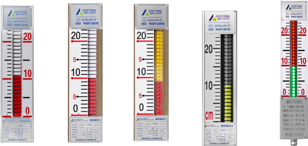
常温面板 中温大刻度面板 高温大刻度面板 不锈钢抽真空面板 磁敏电子双色面板
