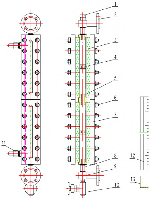
1.放空管帽 2.连接法兰 3.玻璃板玻璃 4.玻璃板芯 5.垫片 6.紧固件 7.压盖 8.连接管 9.三通 10.排污阀 11.保温装置 12.碳钢玻璃板上标尺支架 13.不锈钢玻璃板标尺
