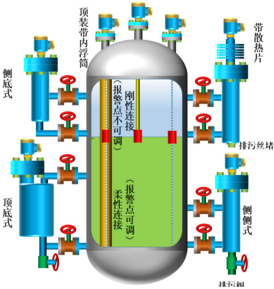
安装示意图
