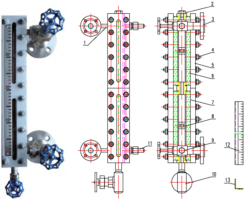
1.连接接头 2.堵头螺丝 3.连接法兰 4.紧固件 5.压盖 6.玻璃板玻璃 7.垫片 8.玻璃板芯 9.考克阀体 10.排污阀 11.保温装置 12.碳钢玻璃板上标尺支架 13.不锈钢玻璃板标尺
