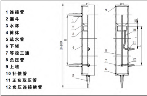
双室平衡容器结构图
