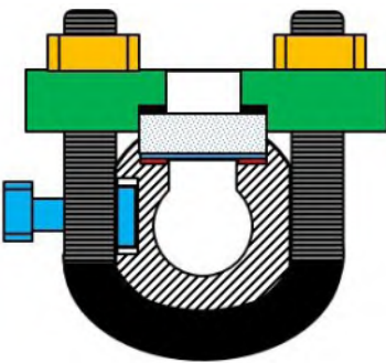
大口径反射式玻璃板液位计
