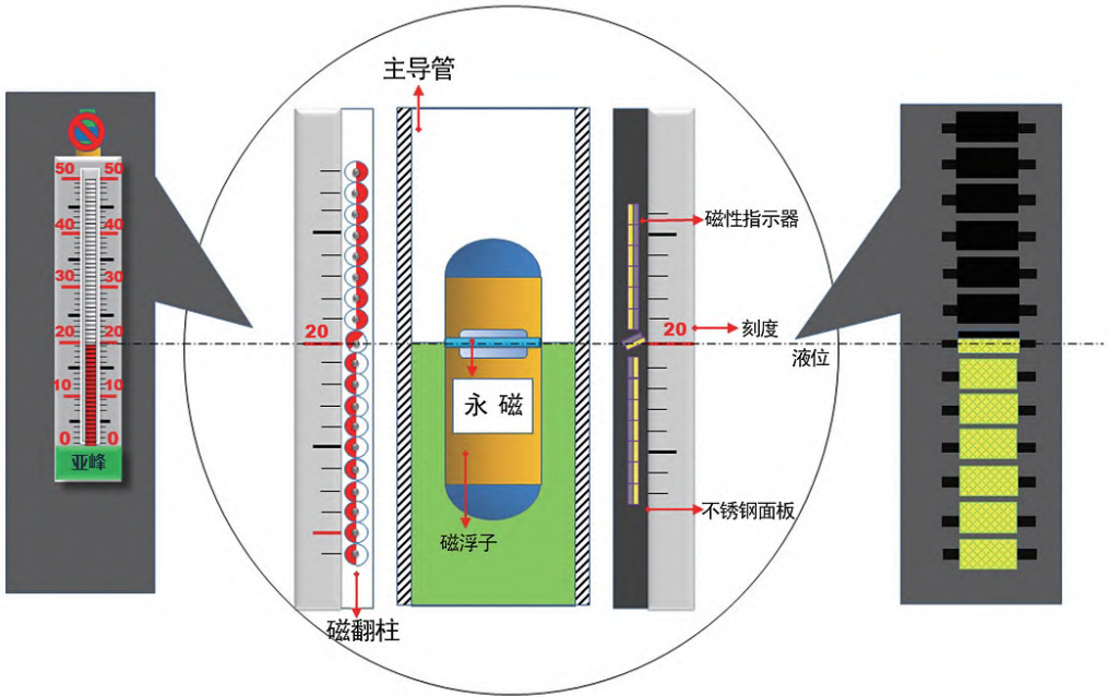
磁性液位计工作原理图
