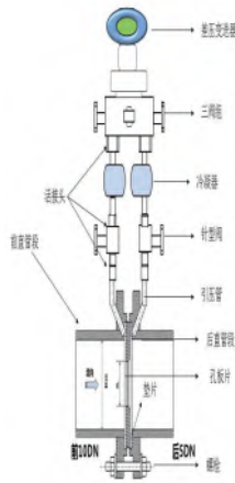
一体孔板装置安装示意图
